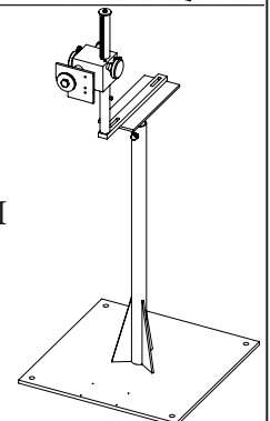
98-0320 XY HEAD ADJUSTMENT ON MINI STAND W/18" BASE
